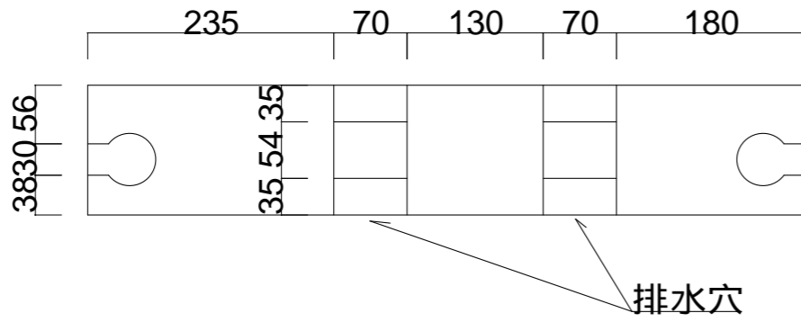
底面図
